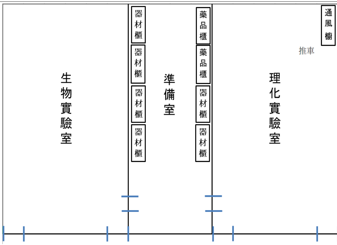
平 面 圖
